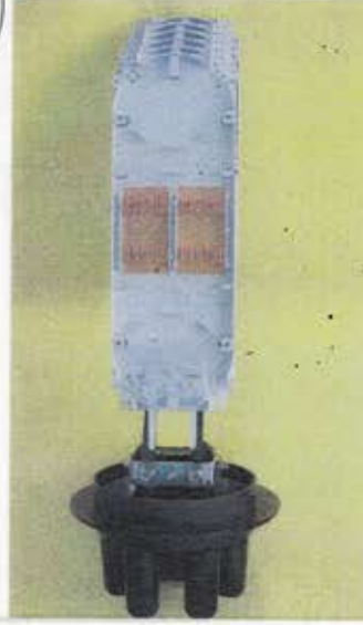
2.1 Fiber Optik Ek Kutusu (İç Görünüm)
